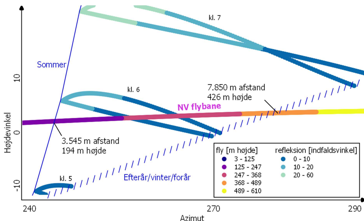
Figur 4 Krydsning af refleksionsstrålen og NV flybane, set fra solcelleparksens centerpunkt. Indfaldsvinkel af refleksionsstrålen på solpaneler er vist
