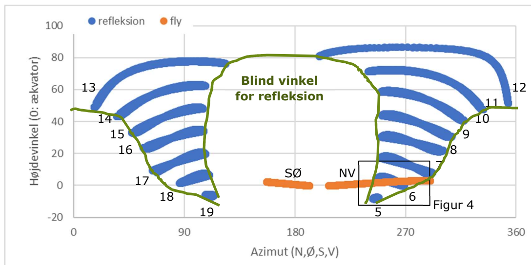
Figur 3 Refleksion af sollys for hele timer i årets forløb (blå) og position af flybane (orange), set fra solcelleparkens centerpunkt. Krydsning af reflekteret sollys og NV flybane er vist med firkant og i Figur 4.
