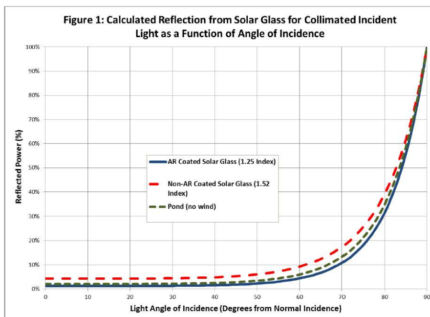
Figur 2 Typisk afhængighed for reflektans fra solpanelglas af sollysets indfaldsvinkel /1/
